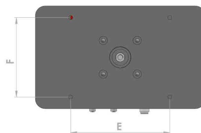
ATSV - piastra di interfaccia
